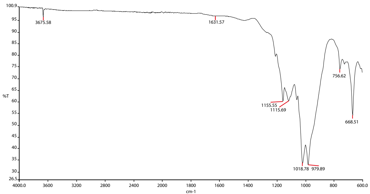
FT-IR RevMix 30
